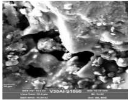
Şekil 5.93 %30 Afşin uçucu kül katkılı Vitriifiye numunelerinin SEM görüntüleri.
