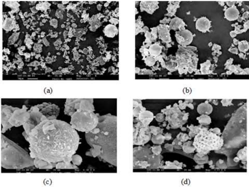
Şekil 4.7 Çayırhan uçucu külünün mikroyapısı, (a) Taneciklerin genel dağılımı (x500), (b) Küresel,yarı-köşeli ve köşeli tanecikler (x1500), (c) Alkal felspat kaplı küreler (x6300), (d) Anhidrit taneciği (x4100).
