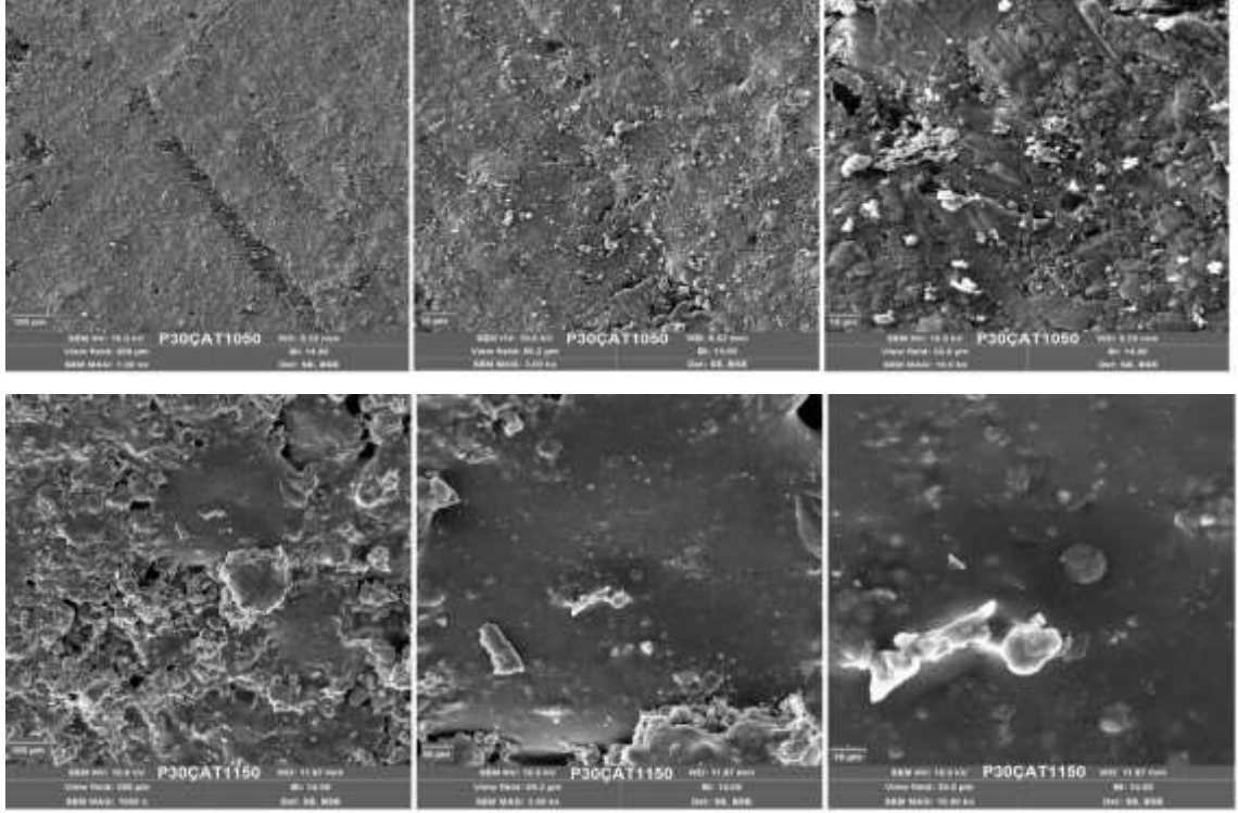
Şekil 5.85 %30 Çatalağzı uçucu kül katkılı Porselen numunelerinin SEM görüntüleri.
