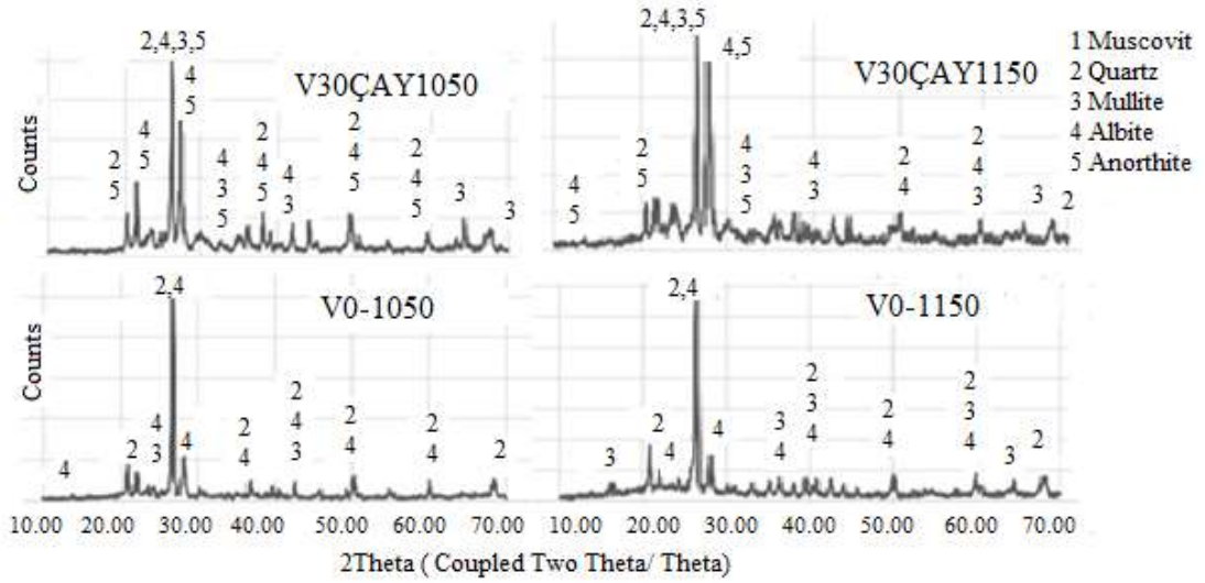
Şekil 5.68 %30 ÇAY katkılı vitrifiye numunelerine ait XRD paternleri.
