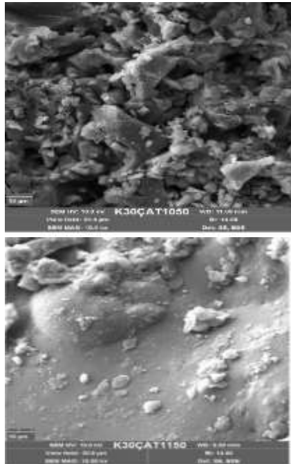
Şekil 5.75 %30 Çatalağzı uçucu kül katkılı Karo numunelerinin SEM görüntüleri.
