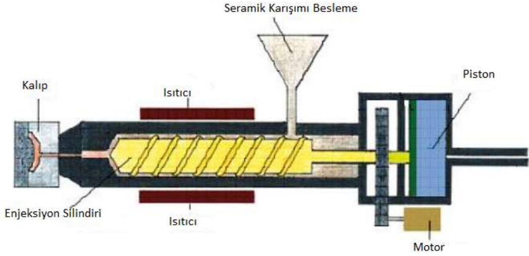
Şekil 3.4 Enjeksiyon kalıpta şekillendirme
