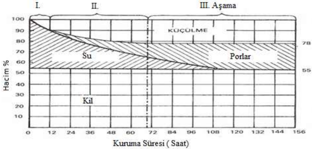
Şekil 3.8. Bourry kuruma diyagramı
