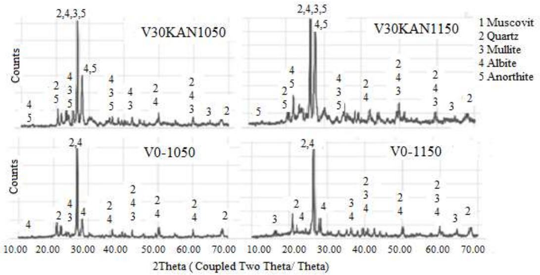
Şekil 5.69 %30 KAN katkılı vitrifiye numunelerinin XRD paternleri.
