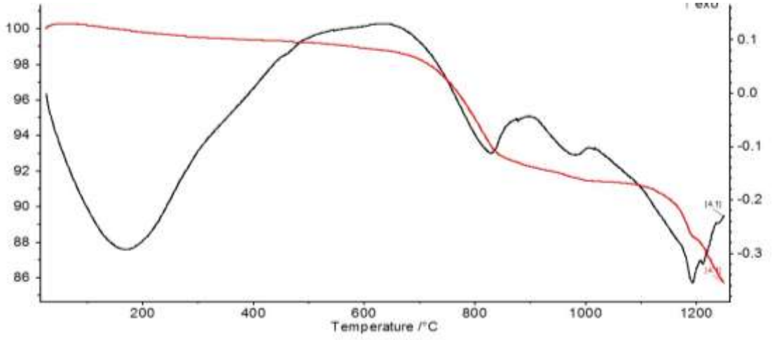
Şekil 4.16 Kangal termik sanrali uçucu külü DTA-TG eğrisi
