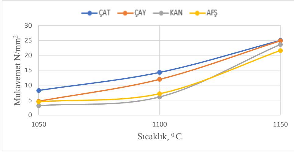
Şekil 5.38 %15 katkı sırlı karo numunelerinin mukavemet – sıcaklık grafiği
