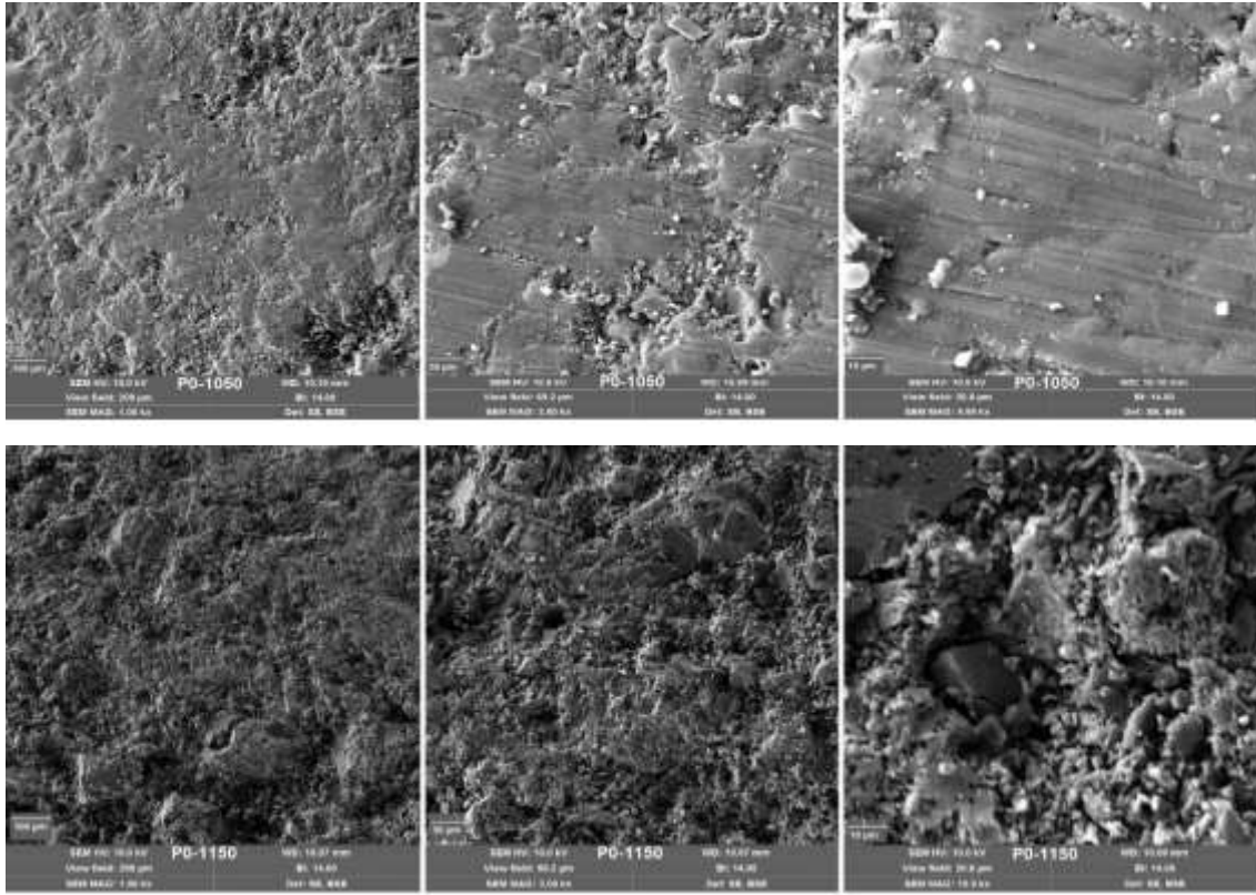
Şekil 5.81 Katkısız Porselen numunelerinin SEM görüntüleri.
