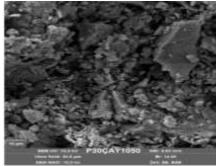
Şekil 5.87 %30 Çayırhan uçucu kül katkılı Porselen numunelerinin SEM görüntüleri.
