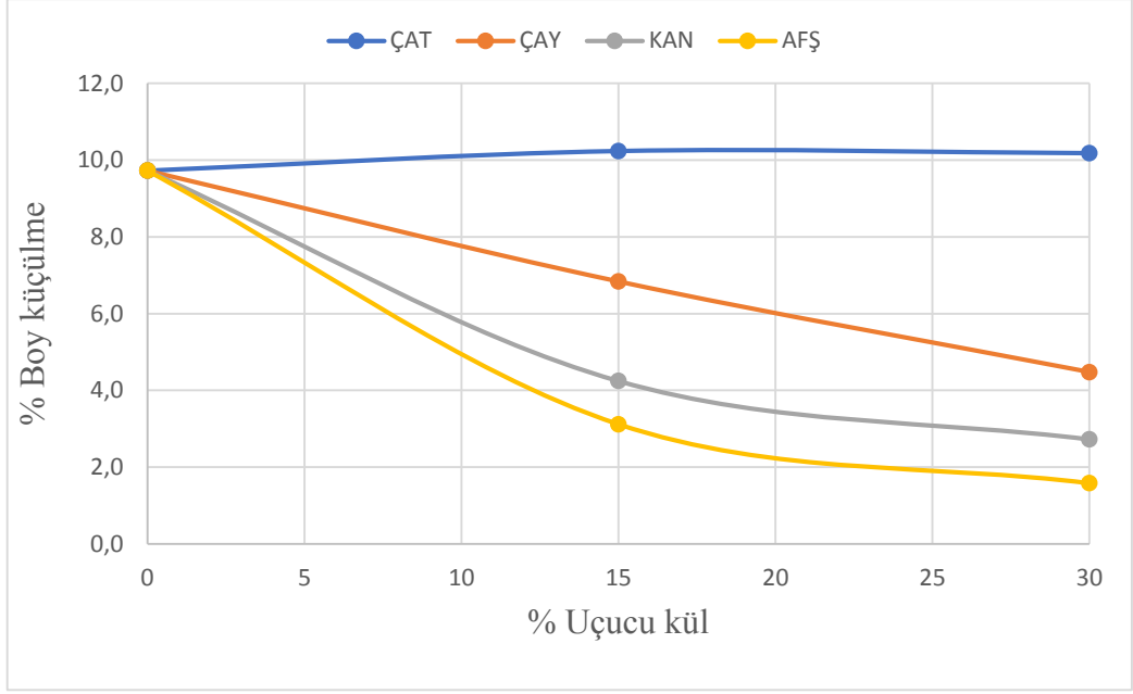
Şekil 5.15 1100 0 C de pişirilen karo numunelerinin uçucu kül- boyca küçülme grafiği
