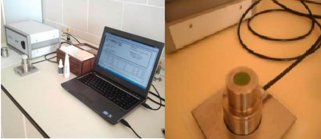
Şekil 4.37 Isıl iletkenlik katsayısı belirleme cihazı (C-THERM / TCi Thermal Conductivity)
