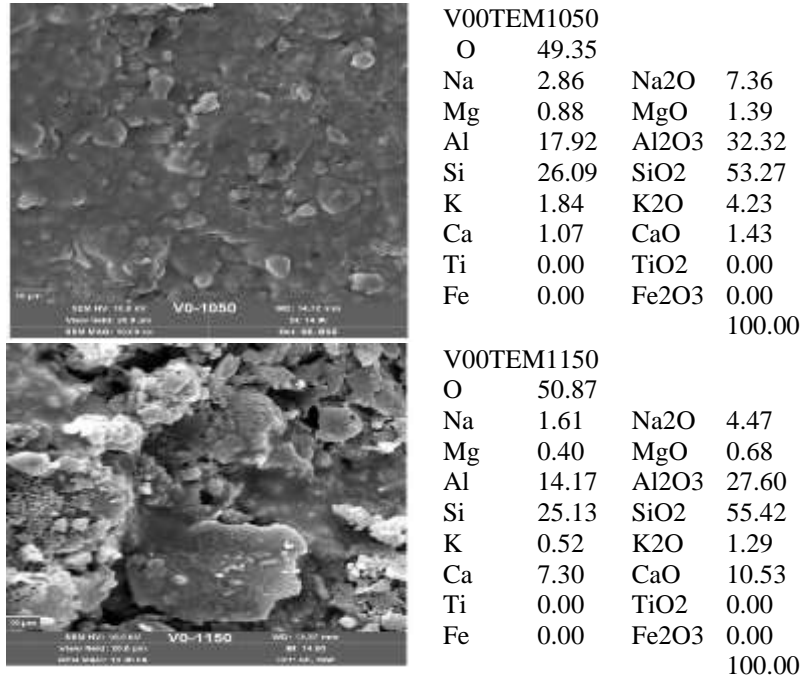
Şekil 5.91 Katkısız Vitrikiye numunelerinin SEM görüntüleri.
