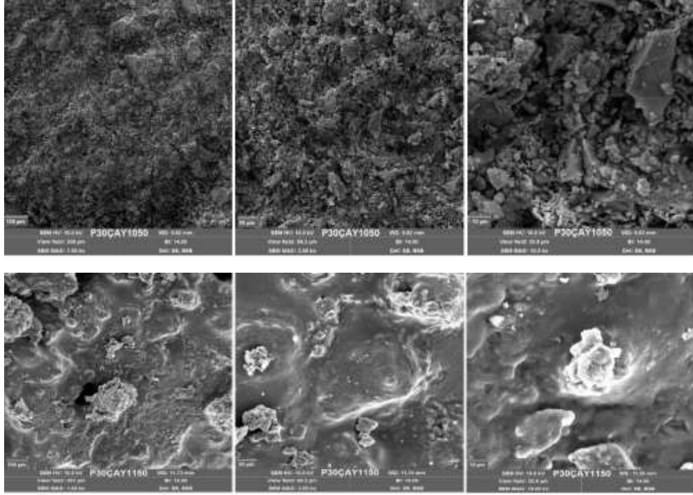
Şekil 5.87 %30 Çayırhan uçucu kül katkılı Porselen numunelerinin SEM görüntüleri.
