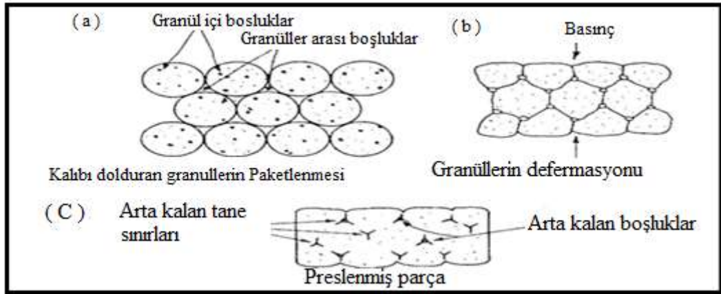
řekil 3.13 Presleme ařamasında granllerin řekil deęiřtirmesinin řematik gsterimi; (a): kalıbı dolduran granllerin paketlenmesi, (b): basın altında granllerin deformatsyonu, (c): preslenmiř para.
