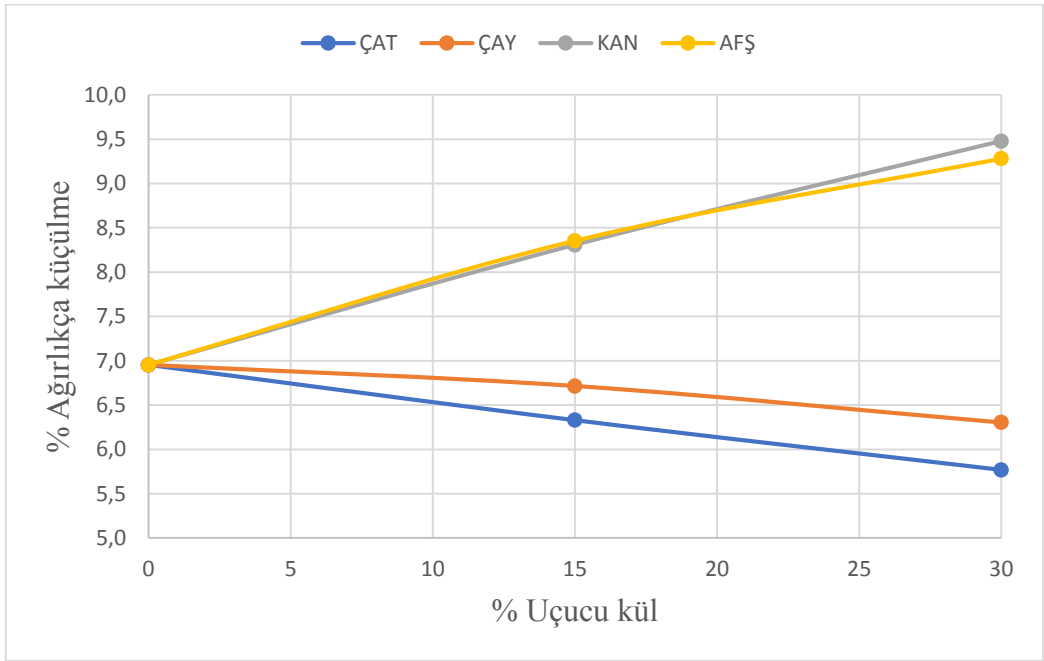
Şekil 5.24 1150 0 C de pişirilen porselen numunelerinin uçucu kül- ağırlıkça küçülme grafiği
