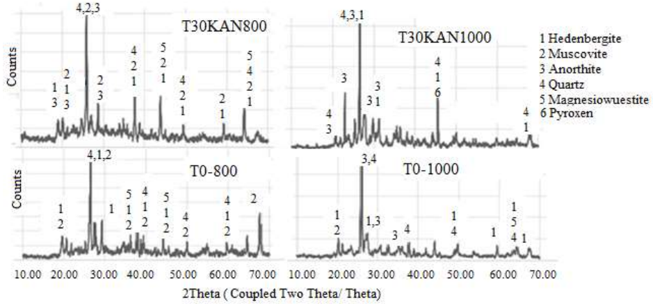
Şekil 5.63 %30 KAN katkıli karo numunelerine ait numunelerin XRD paternleri.
